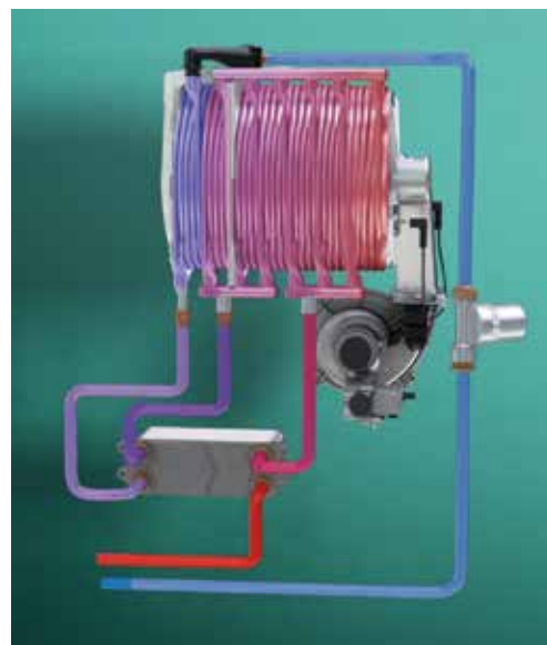
Corps de chauffe extraCONDENS, + 8 % de rendement.
